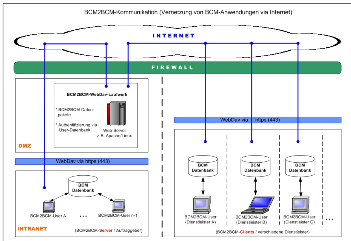
Abb. 6: BCM2BCM - Kommunikation (Schema)
